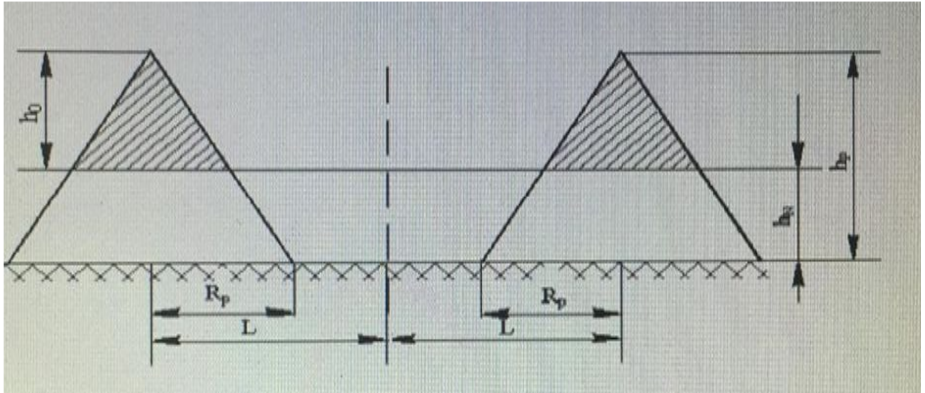
1 сурет- Үйіндіге техникалық рекультивациялаула топырақгрунттарын төгу сұлбасы
